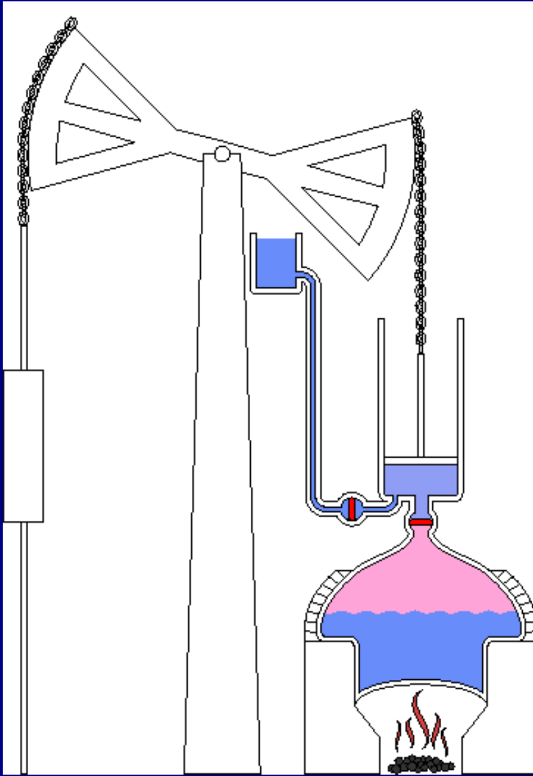
Newcomenův parní stroj 1712
